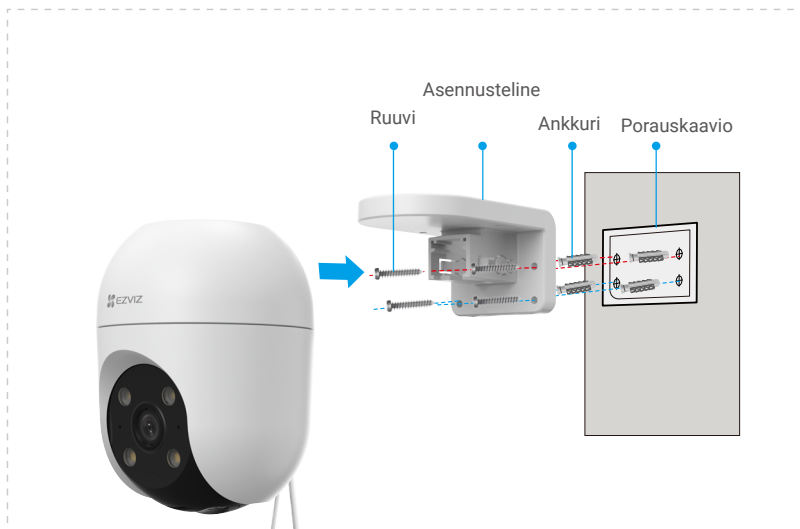
Kuva 2 Seinäasennus
