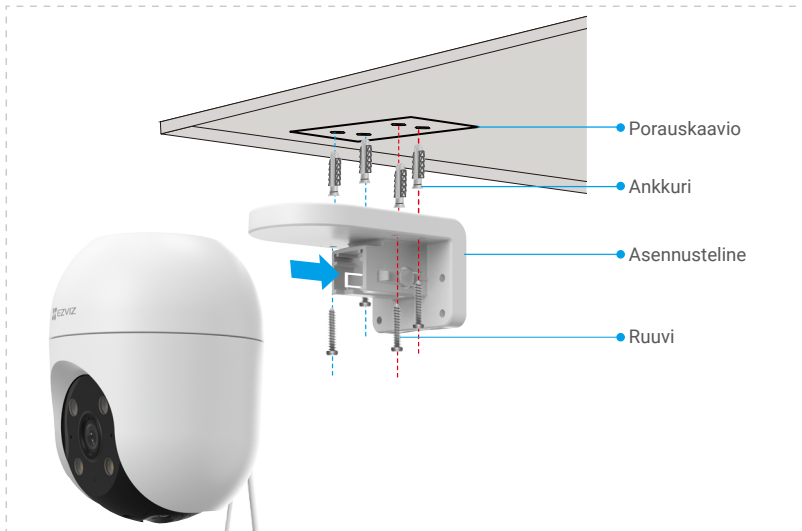
Kuva 1 Kattoasennus
